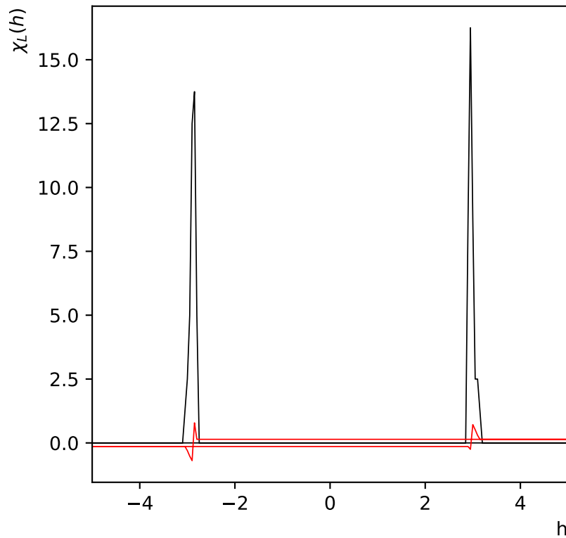
\chi_L(h) réseau de taille L=4 à T=0.5
