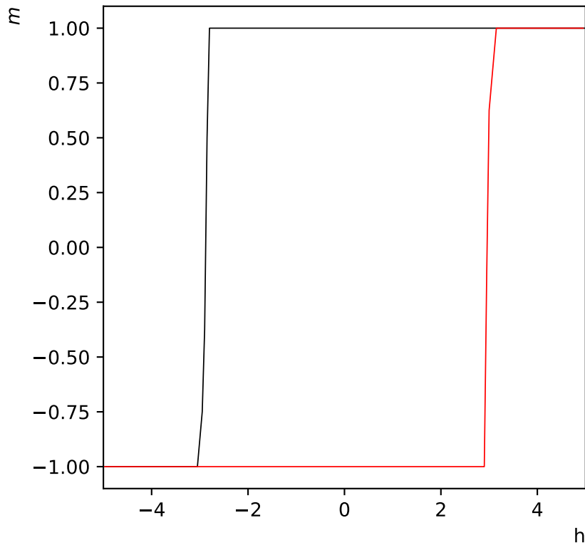
Hystérésis de l'aimantation réseau de taille L=4 - h=5 à T=0.5
